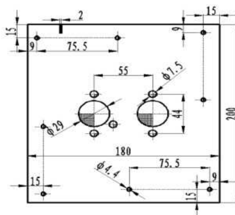
Rys. 10 obrazuje instalację płyty montażowej.
